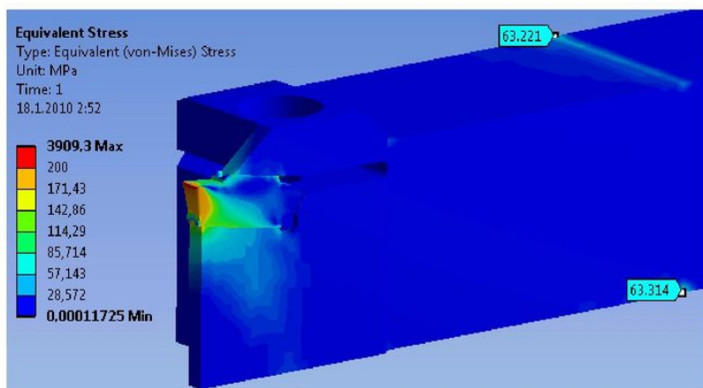
Obrázek 29: Ekvivalentní napětí v nástroji po úpravě stupnice
