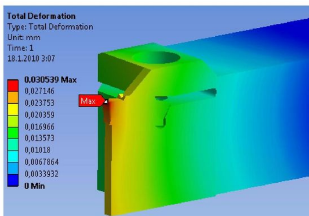
Obrázek 30: Celková deformace nástroje
